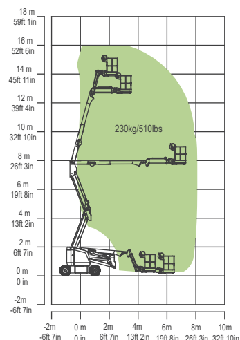
Courbes de travail ZA46JE
