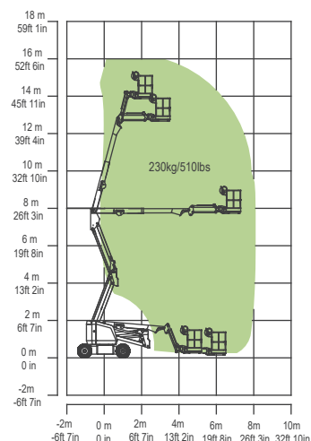
Courbes de travail ZA46JE-Li
